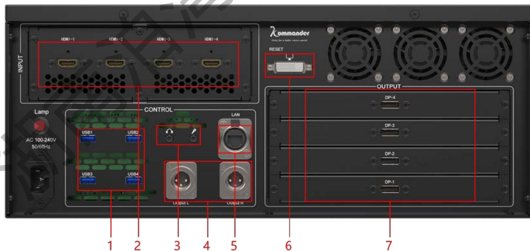
设备背面图
