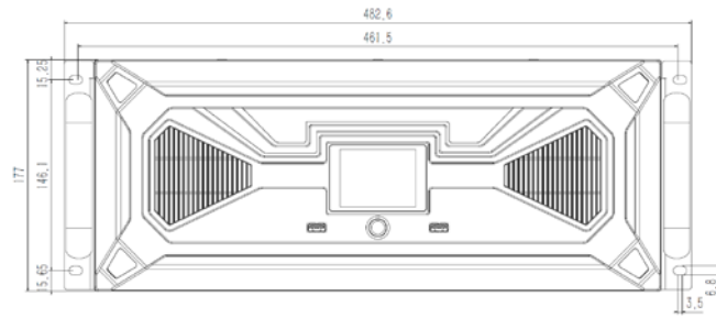
正视图
