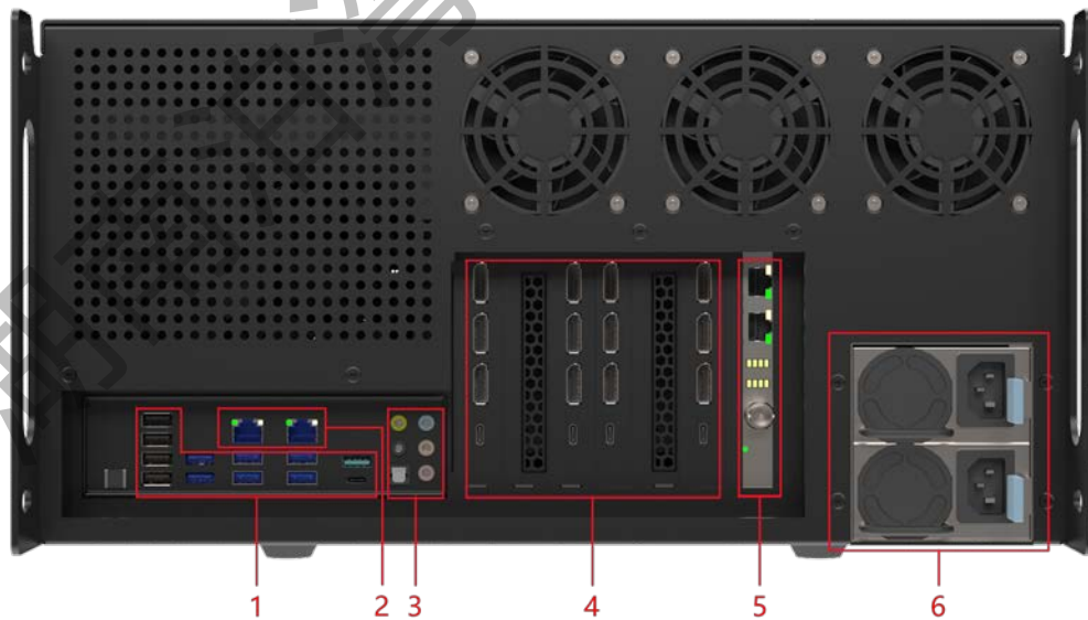
设备背面图
