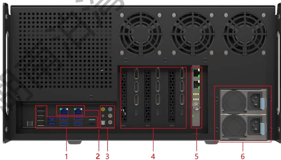
设备背面图
