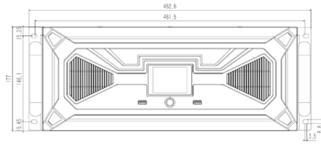
正视图
