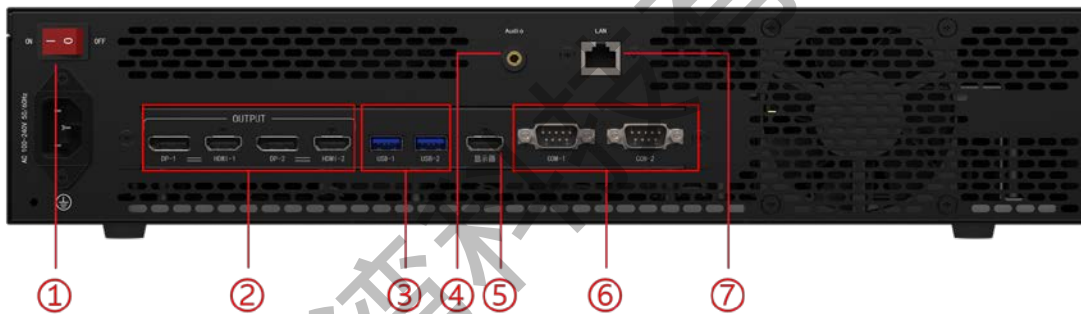
设备背面图
